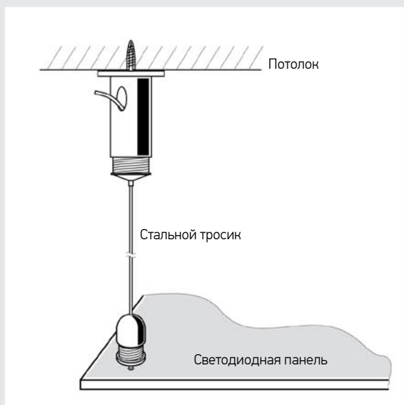
Схема монтажа подвеса PPL A01 4*0.7m
